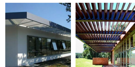
Exemples de brises soleil horizontaux
